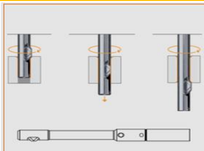
CNC boringontbramer
